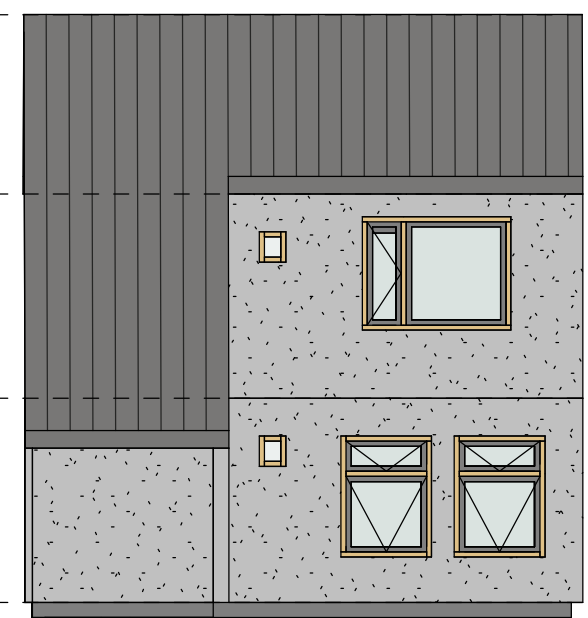
rechtgevel
